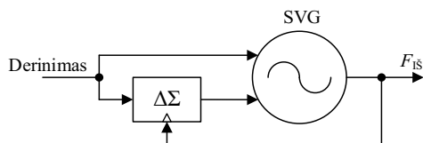
5 pav. Skaitmeniniu būdu valdomas generatoriaus su \Delta\Sigma moduliatoriumi
