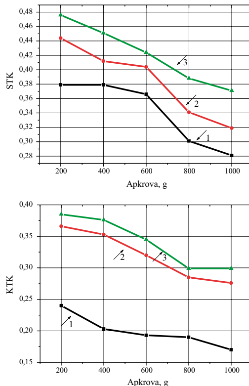
3 pav. Rašaliniai atspaudai, popierius „4CC“. Statinio (STK) ir kinetinio (KTK) koeficientų priklausomybė nuo apkrovos: 1 – popierius į popierių, 2 – popierius į atspaudą, 3 – atspaudas į atspaudą
