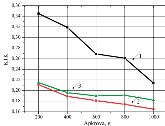
7 pav. Fleksografiniai atspaudai, popierius „4CC“. Statinio (STK) ir kinetinio (KTK) koeficientų priklausomybė nuo apkrovos: 1 – popierius į popierių, 2 – popierius į atspaudą, 3 – atspaudas į atspaudą
