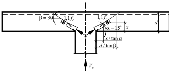
5 pav. Praspaudimo skaičiuojamoji schema pagal Broms (1990) modelį
